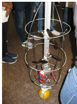
Ferngesteuerte Kegelkugel
